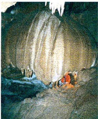
Gouffre du Patu de la Fosse (Arbois).
